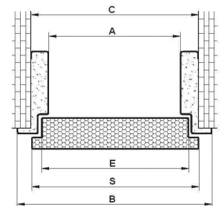
Rysunek poglądowy dla ościeżnic FN, FT SL
