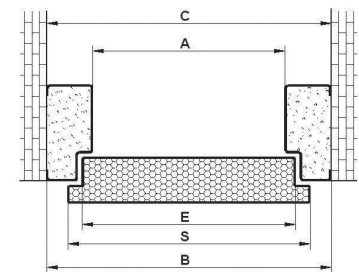
Rysunek poglądowy dla ościeżnic FC, FC SL, FD, FR, FR SL, FA SL
