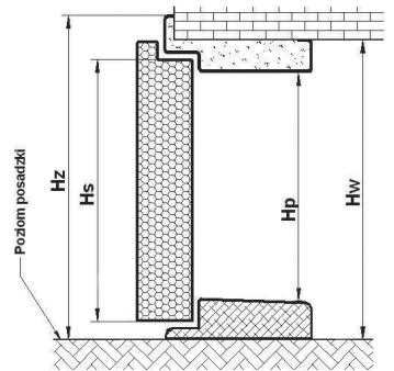
Rysunek poglądowy dla ościeżnic drzwi i progów dla: FN, FN SL
