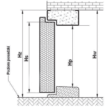
Rysunek poglądowy dla ościeżnic drzwi i progów dla: FD, FC, FC SL, FR, FR SL, FA SL
