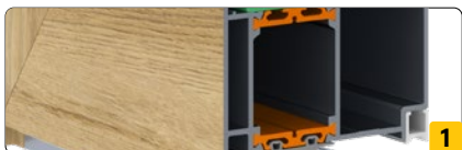
TRZYKOMOROWE PROFILE GŁĘBOKOŚCI 77 MM Z PRZEKŁADKAMI TERMICZNYMI
